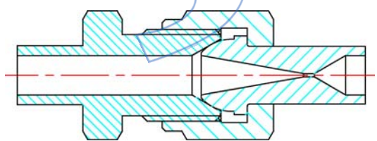
图3 球头密封声速喷嘴组件
