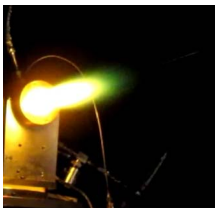
图7 发动机地面热试车照片
