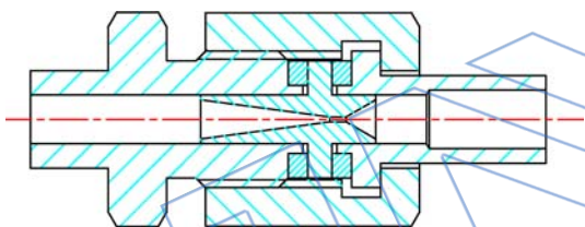
图2 传统声速喷嘴组件
