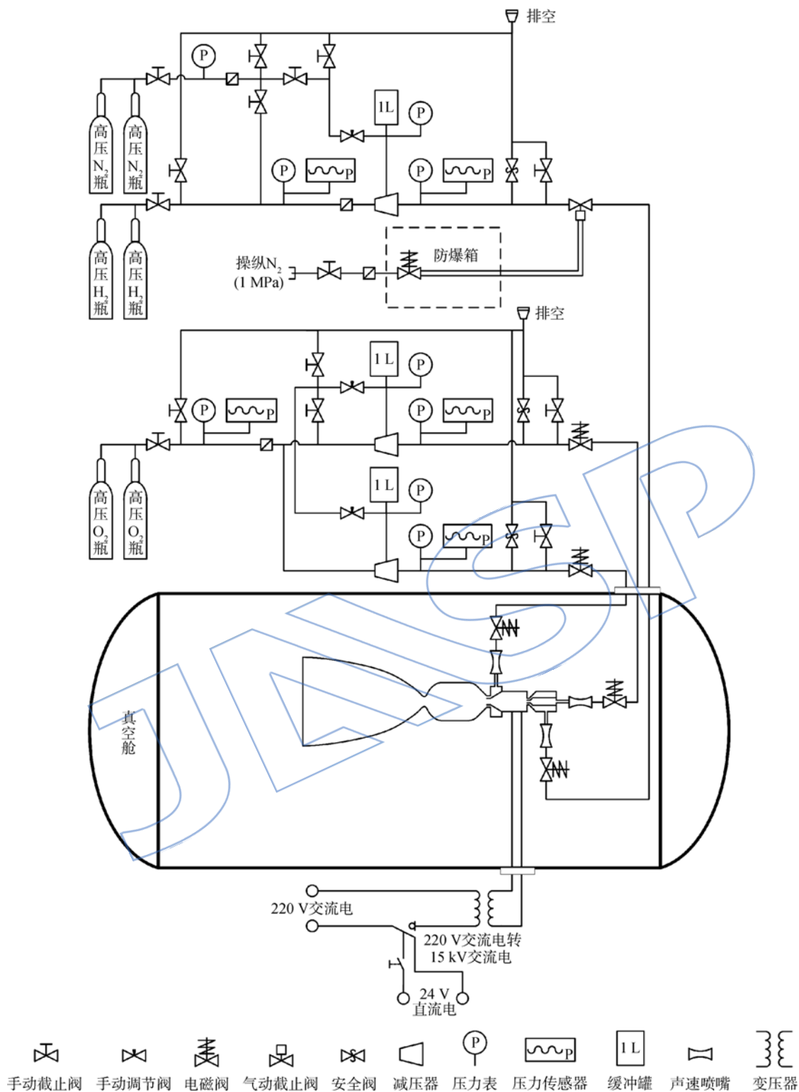
图 6 发动机试验系统原理图
